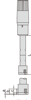
Tip C 12-50mm, karbür ağızlı ölçüm uçları üç ağızlı
