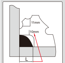
konkav kaynak
