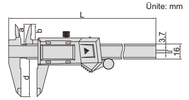
Ünite: mm
