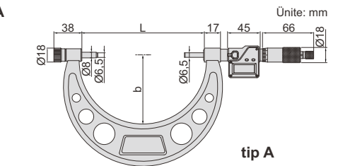
3506-400A
