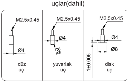
uçlar(dahil)
