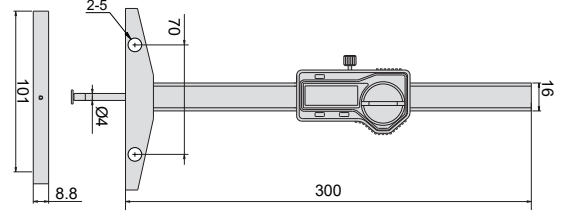
193-006-11 ve 193-008-11
