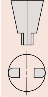
İç çap ölçümleri için oval yüzeyli çeneler
