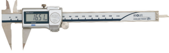
573-621-30 İnce ölçüm çeneli
