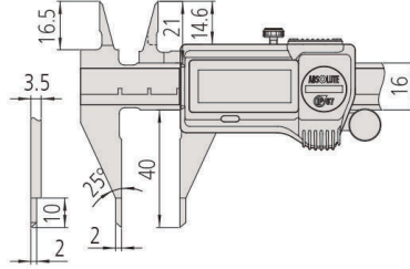
Sivri ölçüm çeneli
