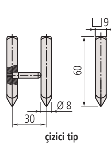
Çizici tip
