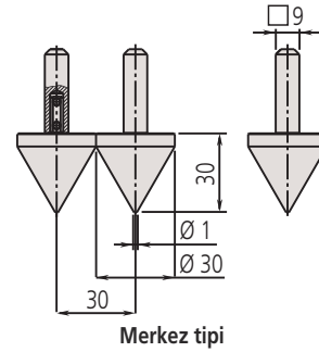
Merkez tipi
