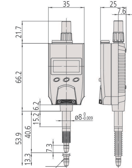
Temas küresi(Ø3) 901312 (dişli:M2,5x0,45)
