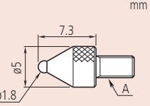
Eklemeli Bilye Uç
