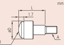
Küresel nokta karbür
