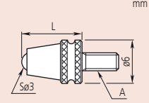
Bilye uç (902119)
