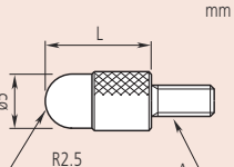
Oval tip uç
