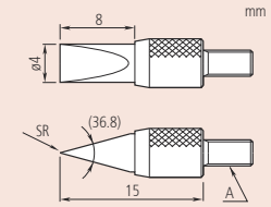
Bıçak ağızlı uç
