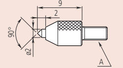
Konik uç karbür (120057D)
