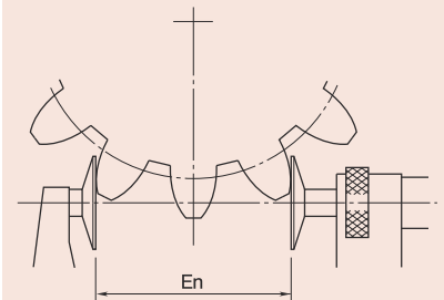
Dişli Teğet Uzunluğu
